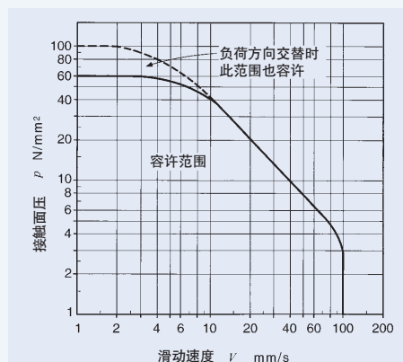
图1 加油式关节轴承的 pV 曲线图
