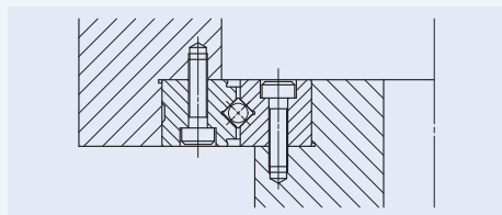
图4 安装在附带安装孔的高刚性交叉滚子轴承(V)的轴承座上的示例
