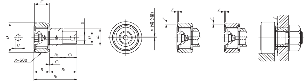
CFE...VBR 偏心轴套外径 d_e 16~41mm
