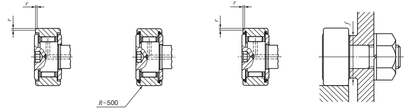
CR...VBR
