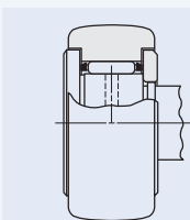
《屏蔽型》
