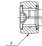
CRH...VBUUR
